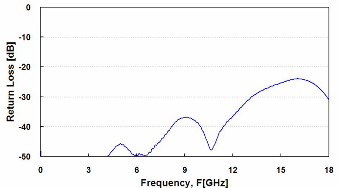
AFS-ADP-AFS BulkHead
